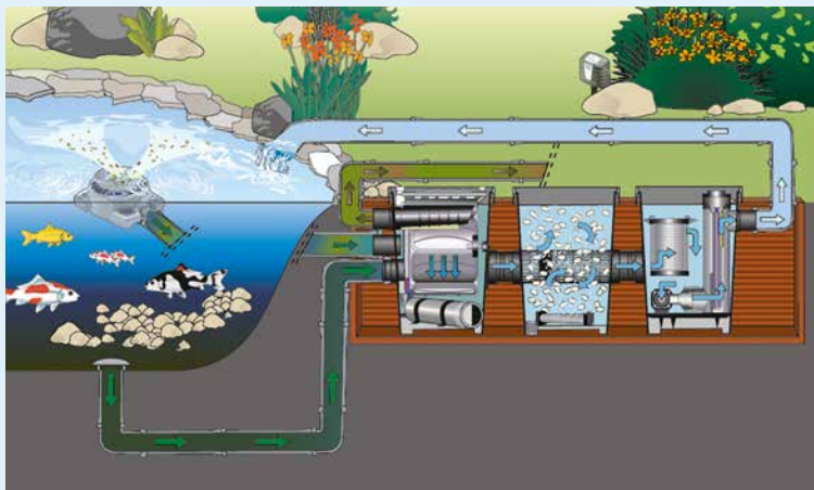
▲ Schematische Darstellung: Gravitationspumpe AquaMax Eco Gravity in Kombination mit den OASE Modulfiltern Proficlear Premium
